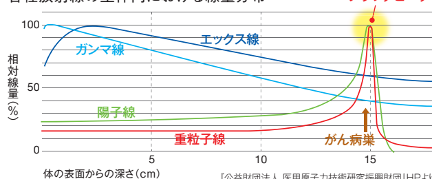
各種放射線の生体内における線量分布
